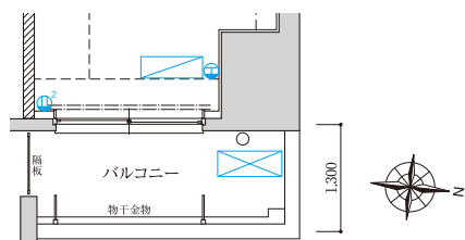
A1 TYPE 部分図
