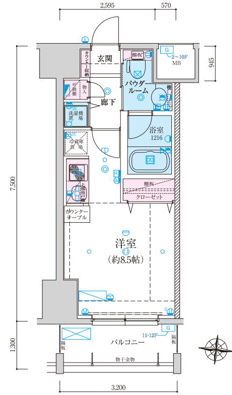
B TYPE 1R 専有面積: 23.96 ㎡(約7.24坪) バルコニー面積: 4.16㎡(約1.25坪)
