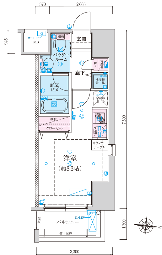
A TYPE 1R 専有面積: 24.03 ㎡(約7.26坪) バルコニー面積: 3.60㎡(約1.08坪)
