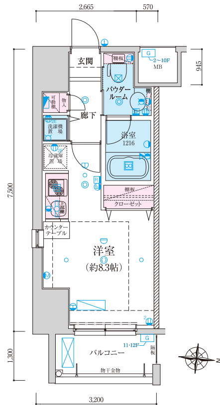
A' TYPE 1R 専有面積: 24.03 ㎡(約7.26坪) バルコニー面積: 3.60㎡(約1.08坪)
