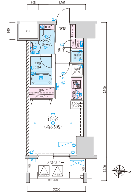
B' TYPE 1R 専有面積: 23.96 ㎡(約7.24坪) バルコニー面積: 4.16㎡(約1.25坪)
